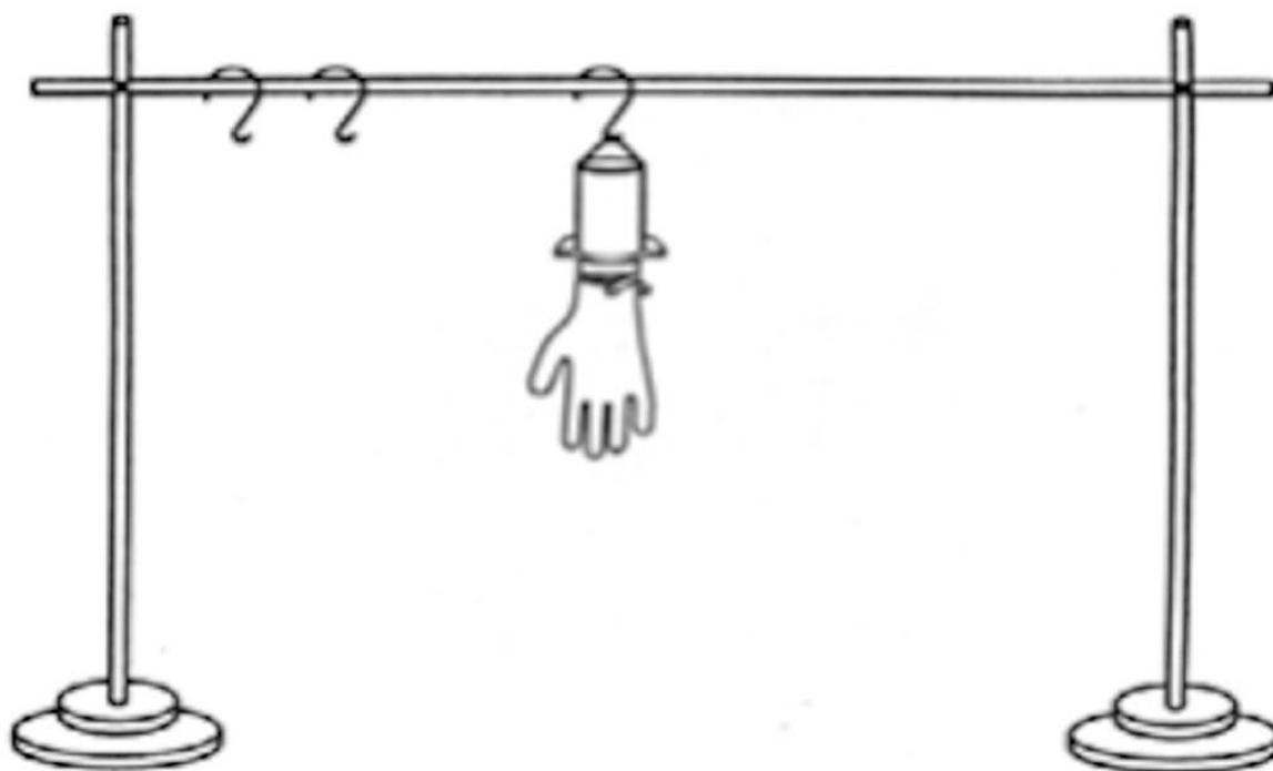
Figura C.2 - Dispositivo de retenção
